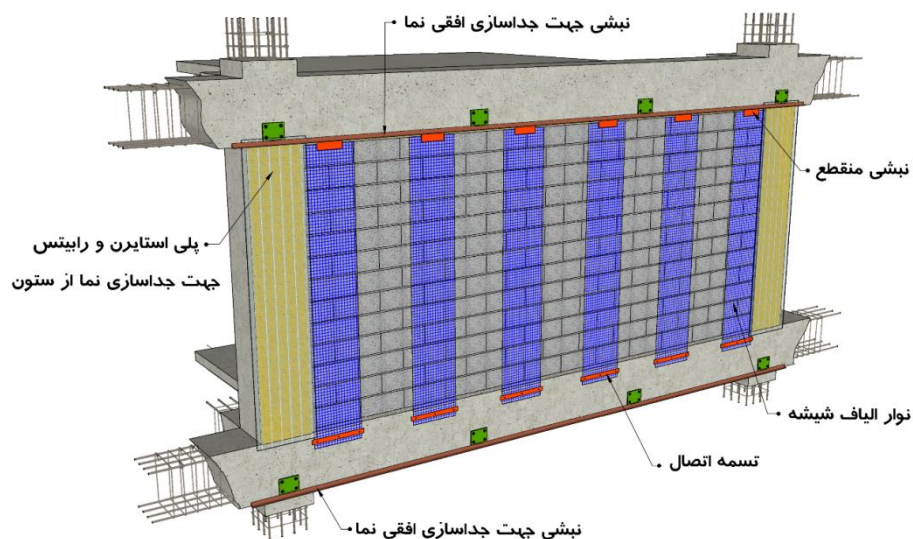
شکل ۳-۱- مسلح کردن دیوارها با استفاده از نوارهای شبکه‌ای الیاف شیشه (سطح خارجی دیوار)
